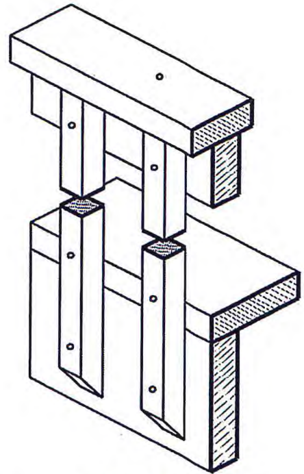
AXONOMETRIC
